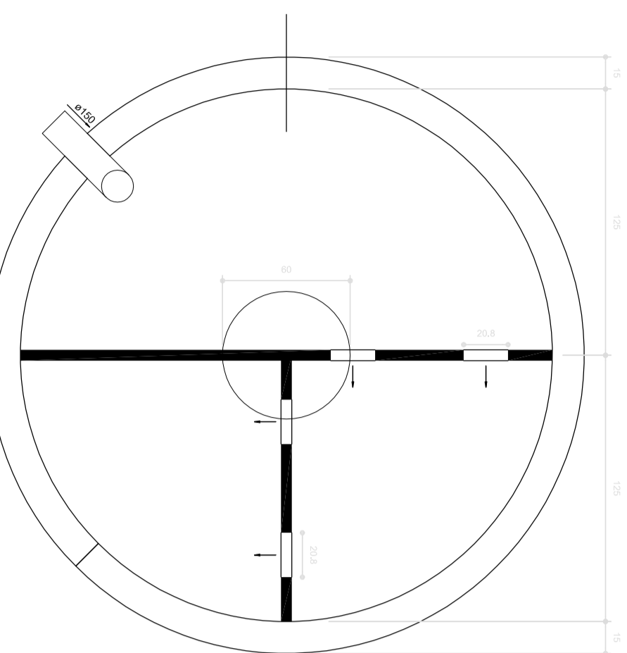
TANQUE SÉPTICO PLANTA BAIXA - ESC. 1:25
